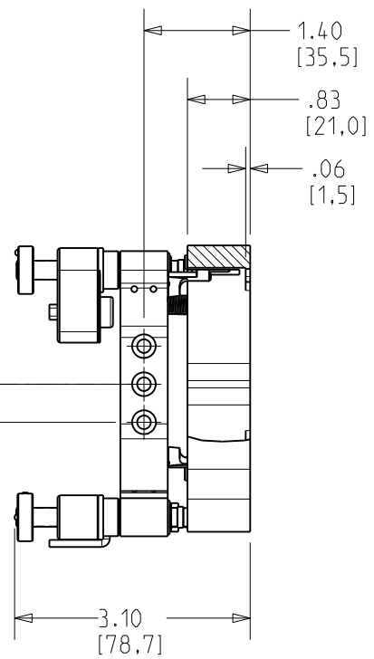
SECTION A-A
