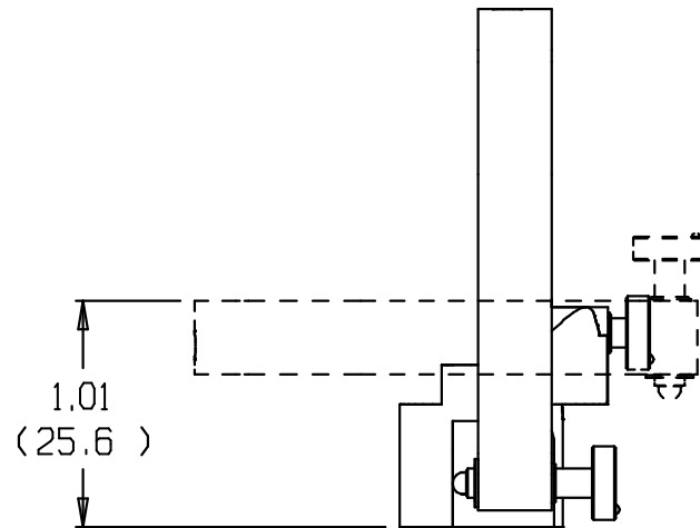
9891-L(M) 1" FLIPPER MIRROR MOUNT
